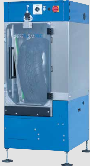
Modulare Waschanlage
